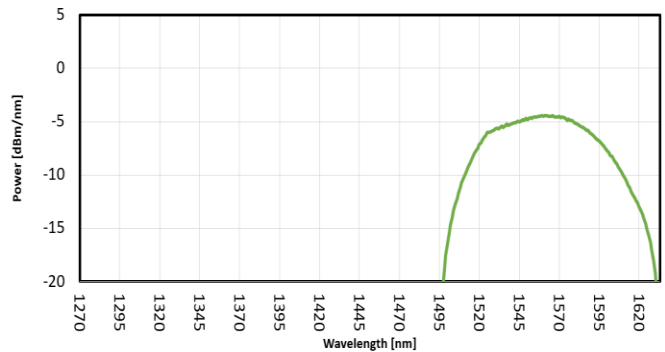
FIG. 2: SLED 1 SPECTRUM
