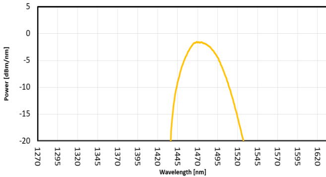
FIG. 3: SLED 2 SPECTRUM
