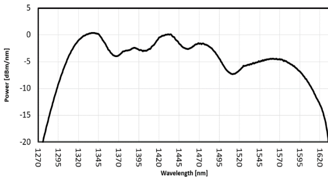
FIG. 1: OSE2 SPECTRUM
