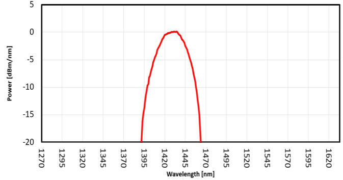
FIG. 4: SLED 3 SPECTRUM
