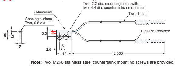
43-G E39-F32A 1M/E39-F32C 1M/E39-F32D 1M
